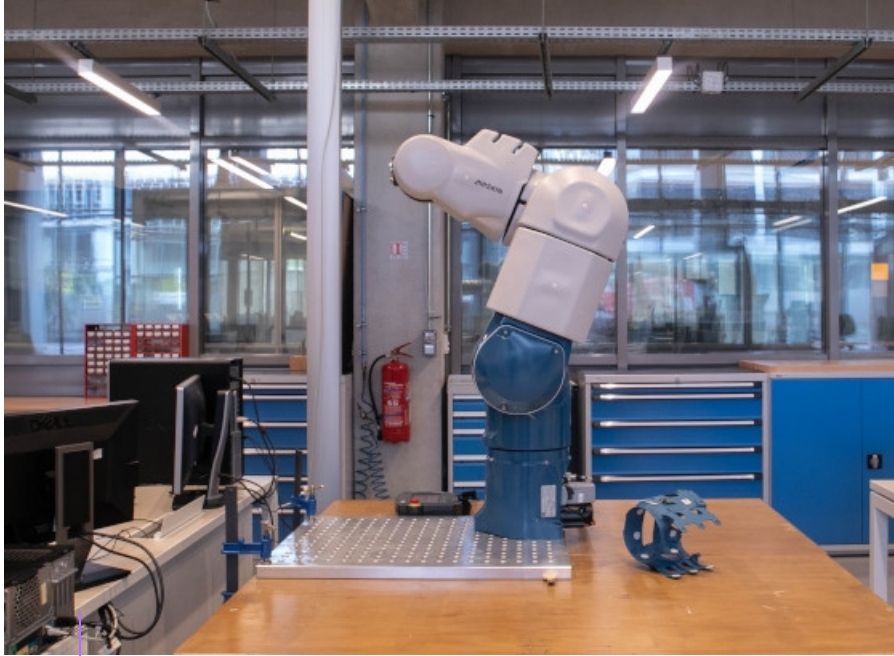
Vue site expérimental - Robot Airskin ©F. DUONG
